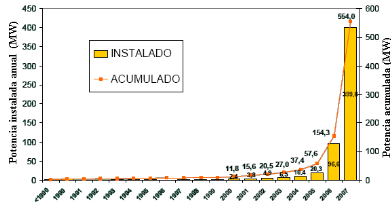
Figura 7.2: Potencia instalada en España hasta 2007.
