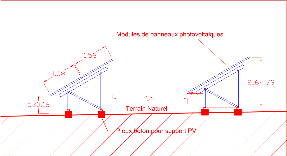
Panneau Photovoltaïque echelle: 1:80
